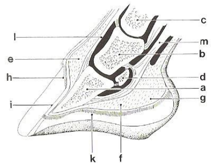
Abb. 6. Längsschnitt durch den Huf des Pferdes
